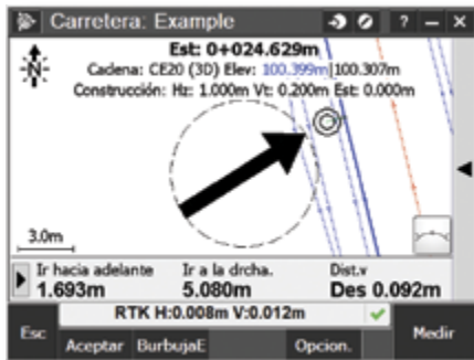
Replanteo por PK en cadena con distancia al eje de construcción horizontal
